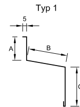
Exempelbild på tröskelbleck.
